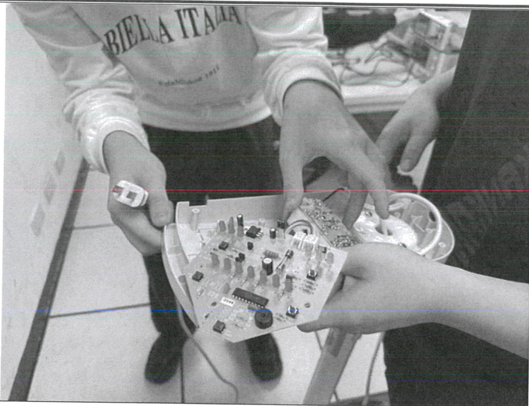
照片 6：電風扇電路板維修檢測
